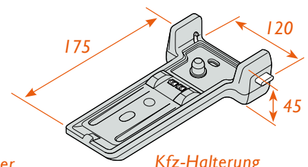
Kfz-Halterung
